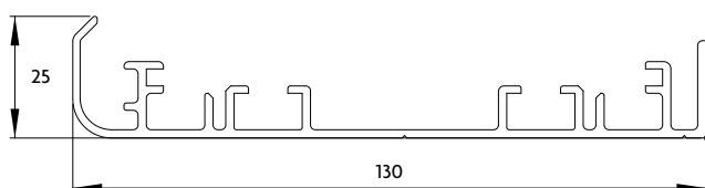
Profilé base
